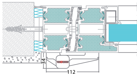
Utenpåliggende hengsele WICSTAR, aluminium
