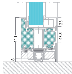
Automatisk heve-/senketerskel (røyktett)
