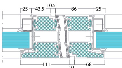
Snitt pardør
