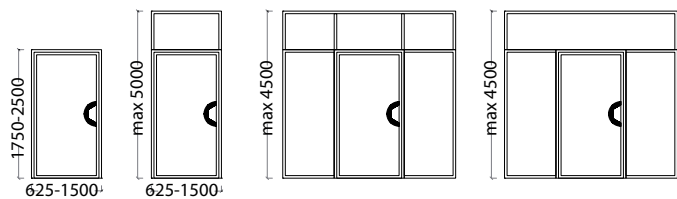
EI90-1 Dør
