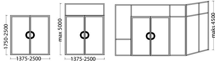
EI90-2 Pardør
