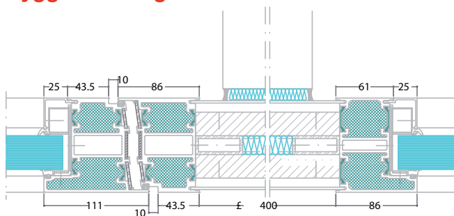
T-anslutning av innervegg
