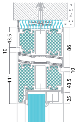
Dørkarm
