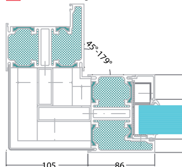
Dør med sidelys / 90* hjørne
